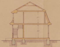
Lõige C.D.
