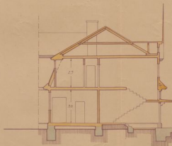
Lõige A.B.
