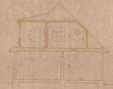
LÕIGE A-B
