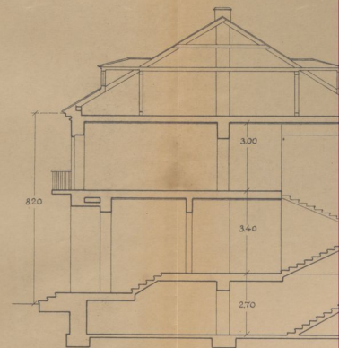
LÕIGE A-B.
