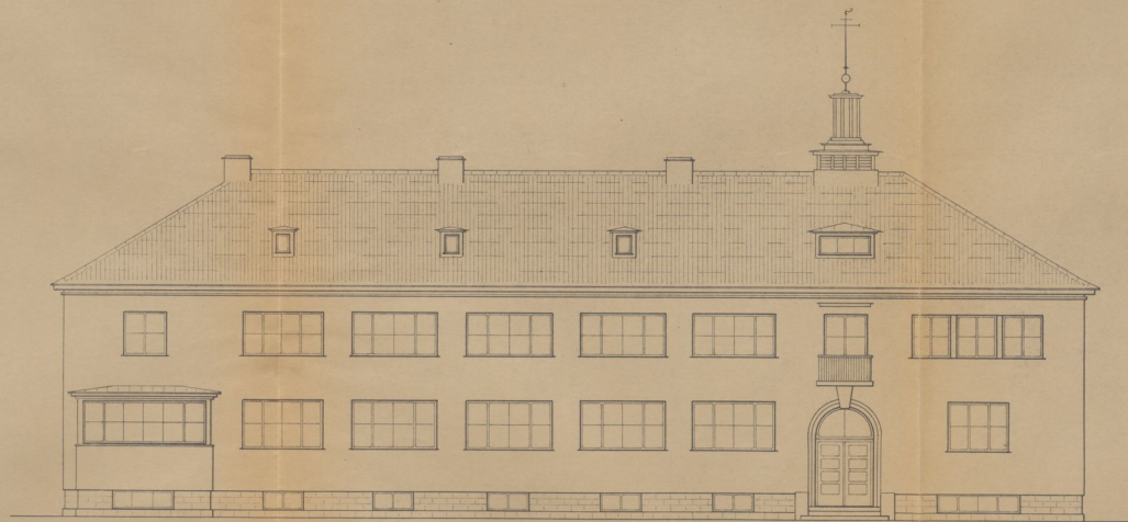
TEEPPOOLNE VAADE.
