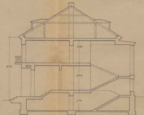
LÕIGE A-B.
