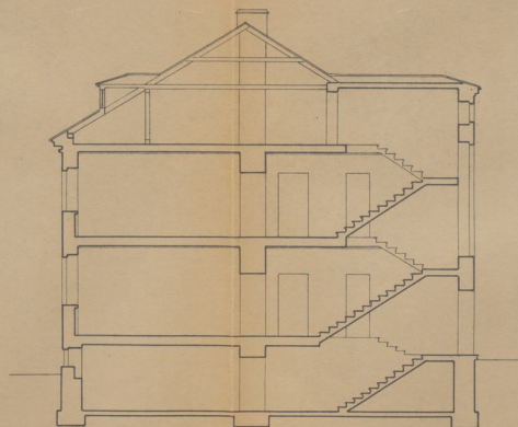
LÕIGE C-D.
