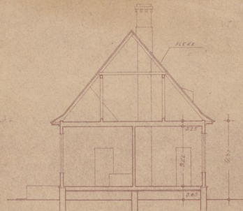
LÕIGE D-E VÄLISEINTE TÄRIND + ASUTAJALISE + LAOPOODK.
