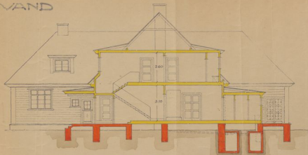
TREPIKOJA LÖIGE
