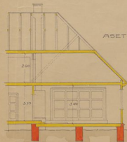
SAALI LÖIGE
