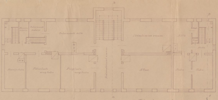
Teine korrus
