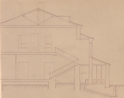
Lõige AB
