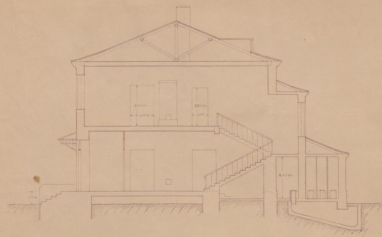
Lõige AB
