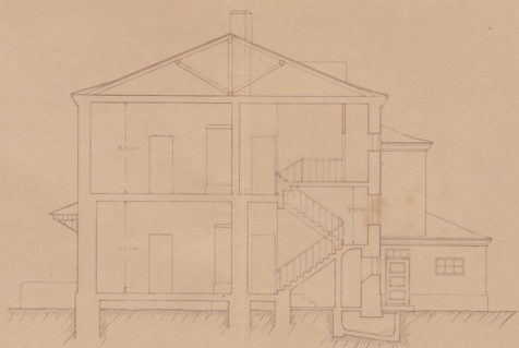
Lõige CD
