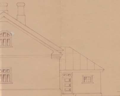
Külvavaade
