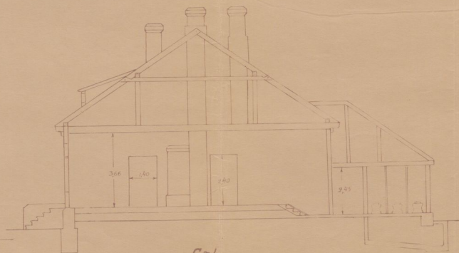
Lõige
