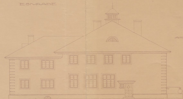
OTSIVAADE
