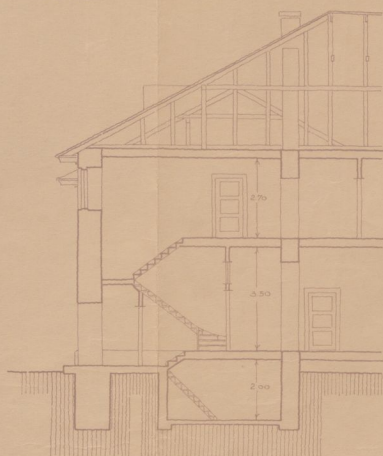
LÕIGE I
