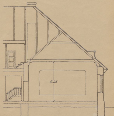
Lõige: 3
