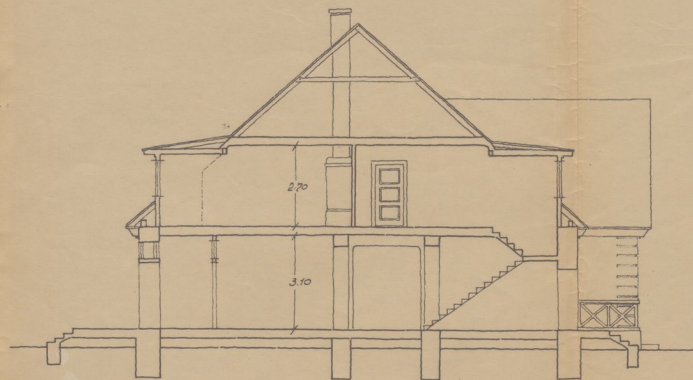
Lõige: 1+2
