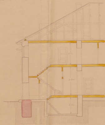
LÕIGE I
