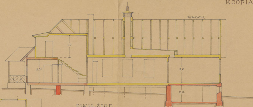
PIKILÕIGE.
