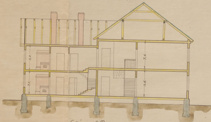
Lõige, A-B.
