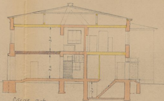
Løise a-b
