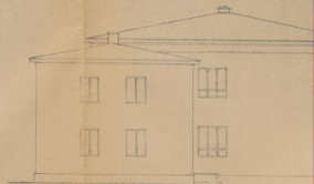
Otsivaade (edelist)
