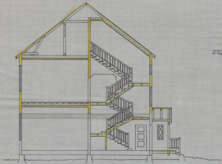
Lõige A-B
