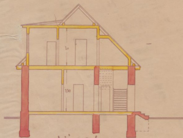
Lõige e-f.
