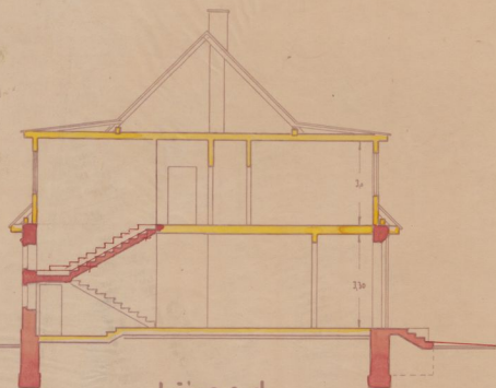
Lõige c-d.
