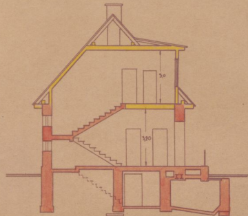
LÖIGE A-B.
