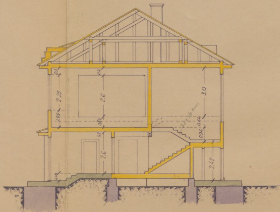
• LÖI GE "A·B" •
