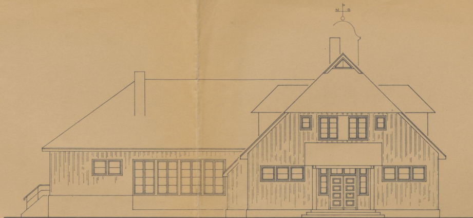
PÕHJA-LÄÄNE VAADE
