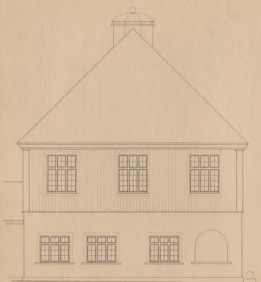
Γόλφο C-C
