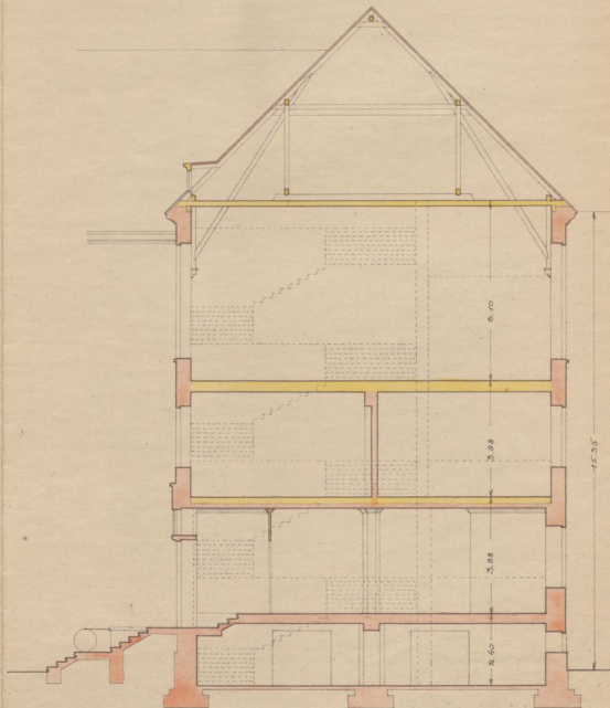
Lõige A-B.
