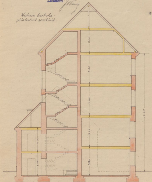
Lõige C-D.
