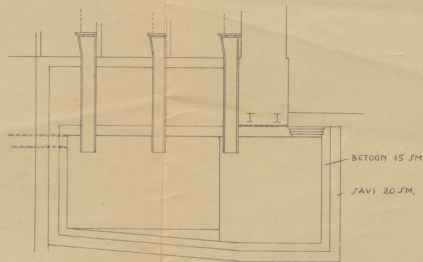
LÕIGE KLOSETI KAEVUST 1:50.
