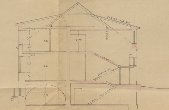
RISTLOIGE A-A
