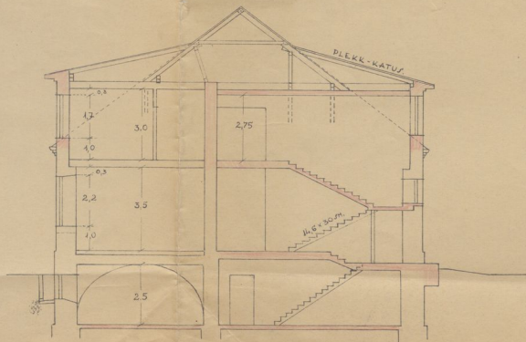
RISTLÕIGE A-A
