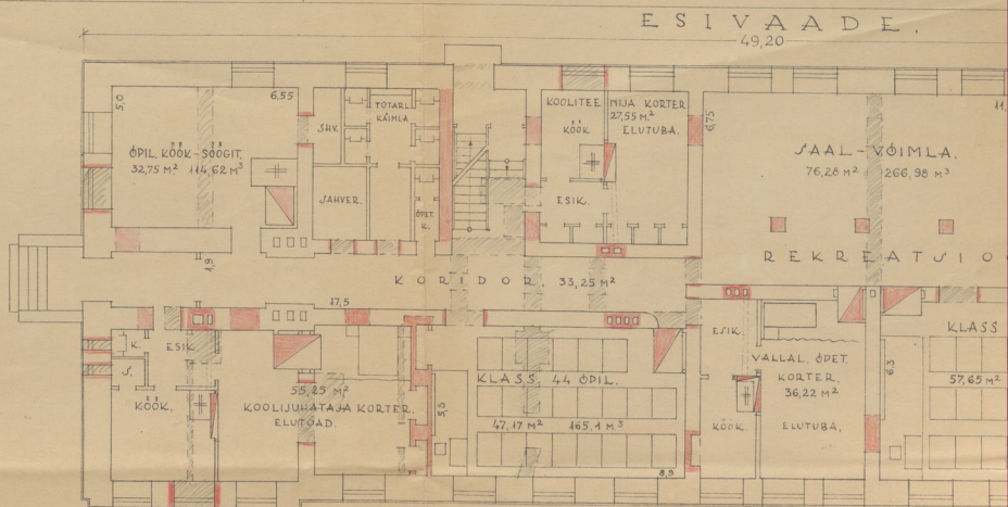
ALUMISE KORRA PLAAN.
