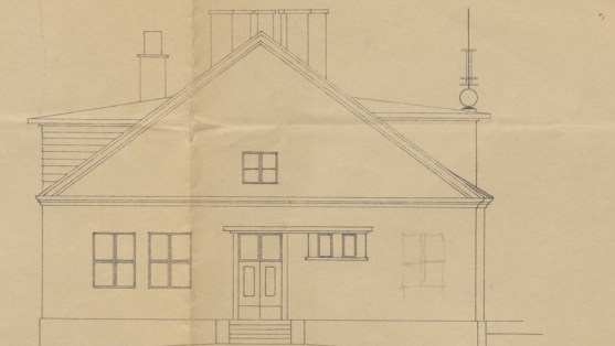
OTSAVAADI.
