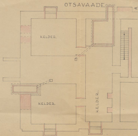
KELDRIKORRA PLAAN.
