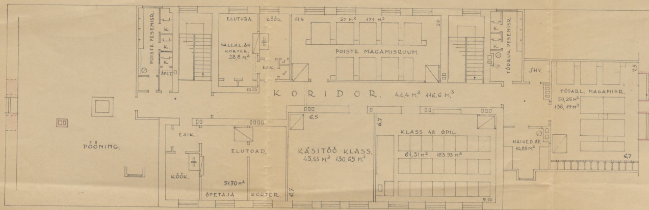
ÜLEMISE KORRA PLAAN.
