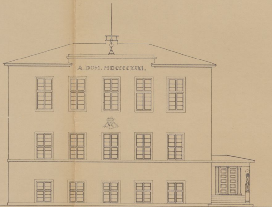
LÄÄNEPOOLNE FASSAAD.
