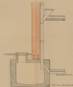
LÖIGE C-D 1:50.
