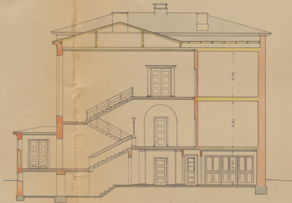
LÖIGE A-B.
