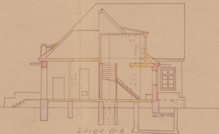
Lõige a-b
