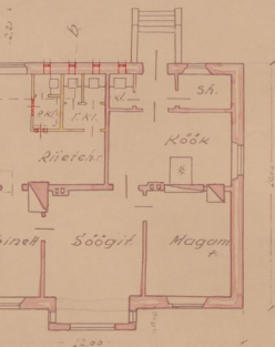
Põhiplaan
