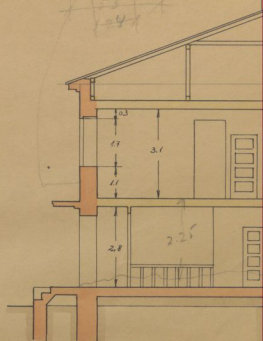
Lõige a-b
