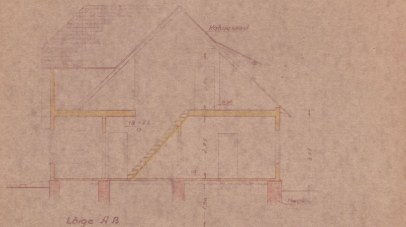
Lõige R.B.
