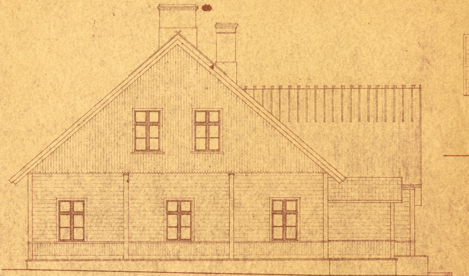
OTSAVAADE
