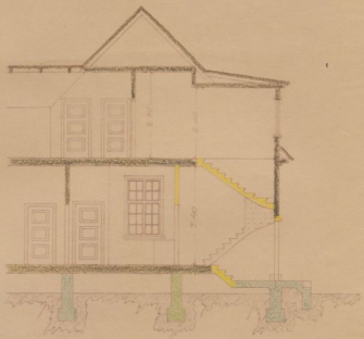
Läbilõige B-B
