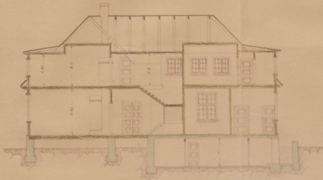
Läbilõige A-A
