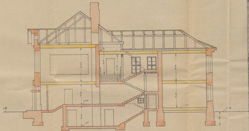
Lõige "A-B"
