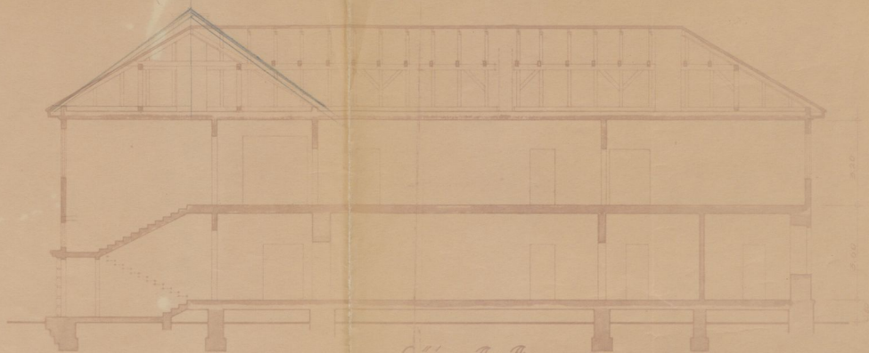
Corte A-A.
