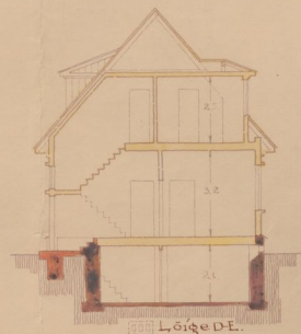
Lõige D-E.
