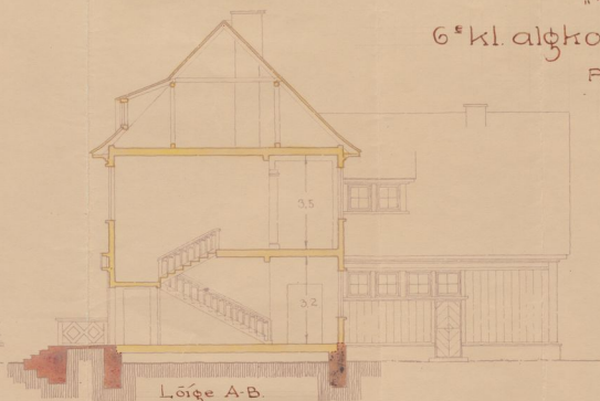
Lõige A-B.
